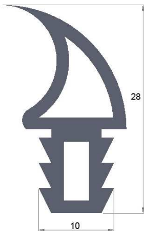
QX283 Silikonski profil 10x28
