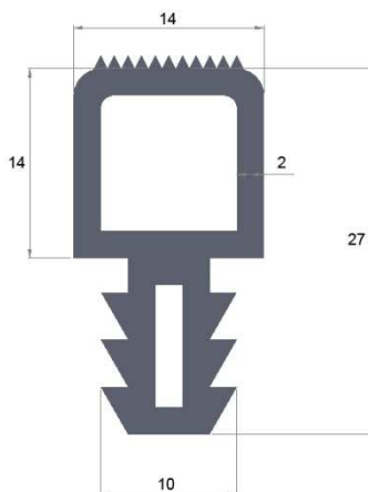
QX271 Silikonski profil 10x27
