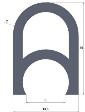
QX139 Silikonski profil "A" 13,5x19
