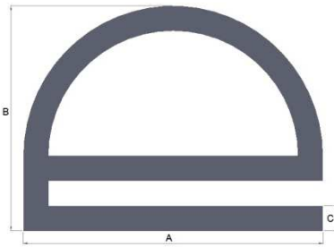
NN003 Sunder ram za vibro sito 80x200x15
