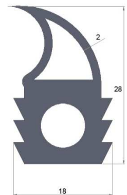
QX282 Silikonski profil 18x28
